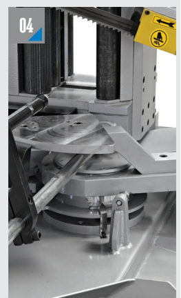
DÖNER GÖBEK SİSTEMİ MITER CUTTING
